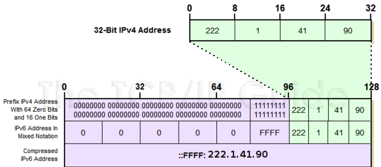
Figura 2: IPv4 mapeada a IPv6
