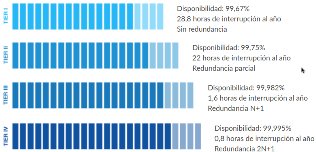
Figura 17: Resumen de niveles TIER
