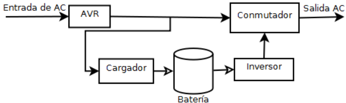
Figura 46: SAI offline interactivo
