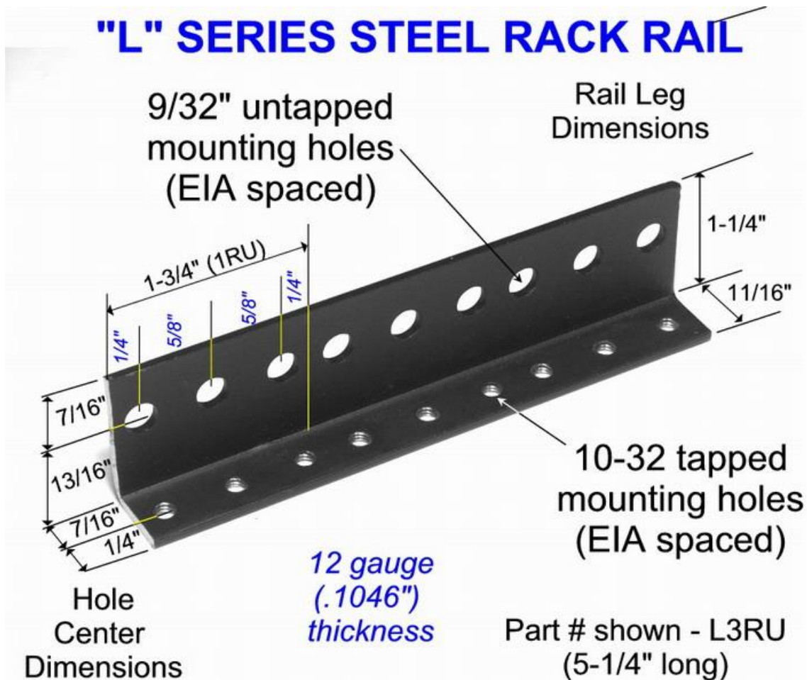
Figura 19: Dimensiones de los railes de un rack
