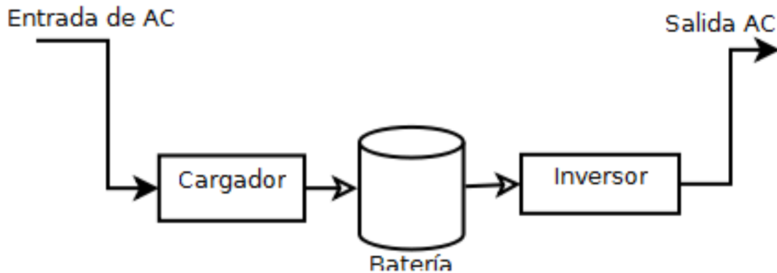
Figura 47: SAI online
