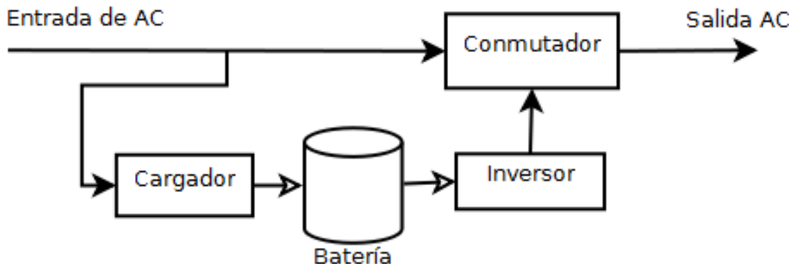
Figura 45: SAI offline
